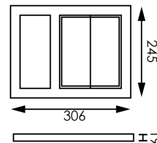
COPERCHIO
